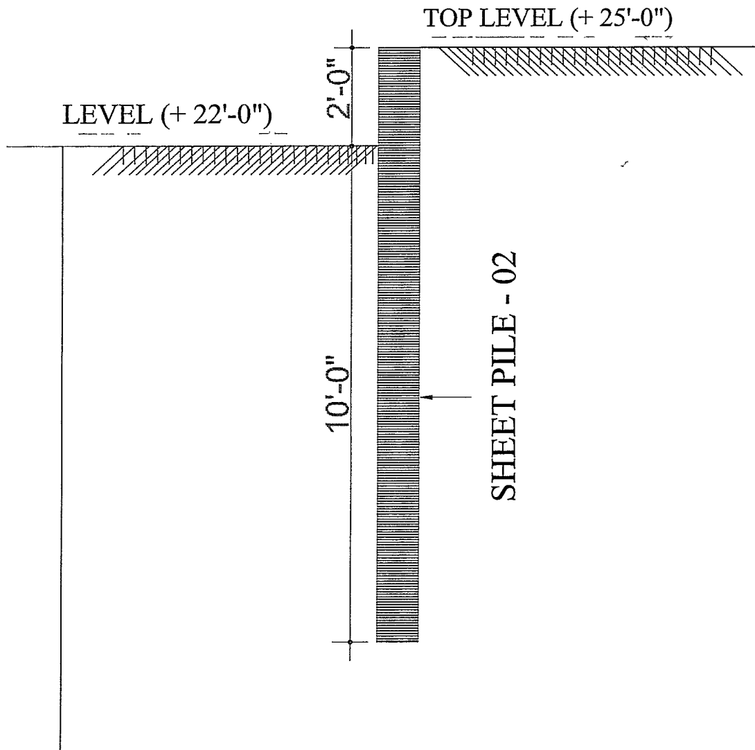
FIG: SHEET PILE -02 ELEVATION
